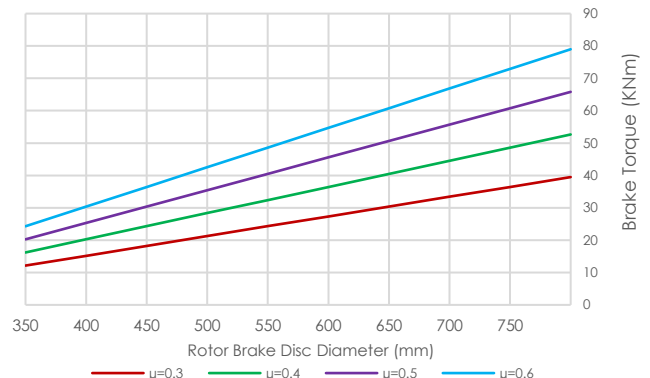
Brake Torque HAB-4-90 RS (P=16Mpa)
